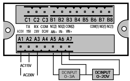
端子盤接線
